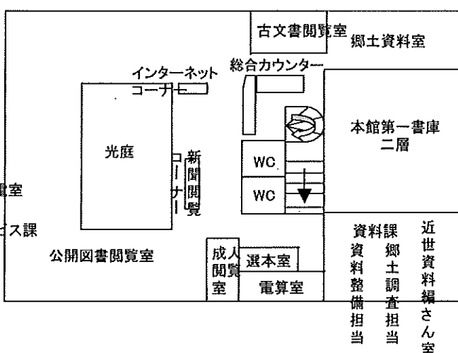
二階平面図
